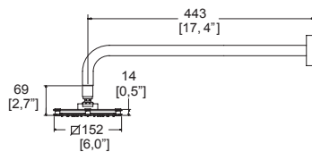
Dimensiones: vista lateral
