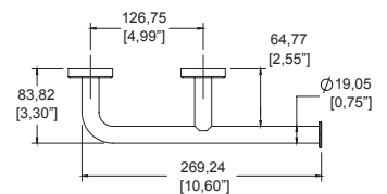
Dimensiones: vista cenital
