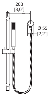
Dimensiones: vista frontal
