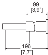
Dimensiones: vista lateral
