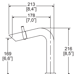
Dimensiones: vista lateral
