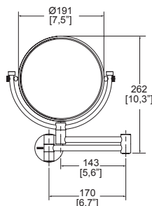
Dimensiones: vista frontal
