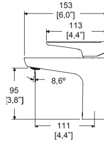
Dimensiones: vista lateral
