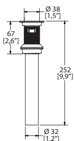
Dimensiones: vista lateral
