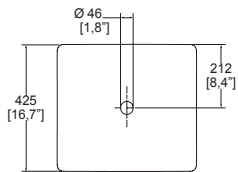
Dimensiones: vista cenital
