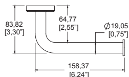
Dimensiones: vista cenital
