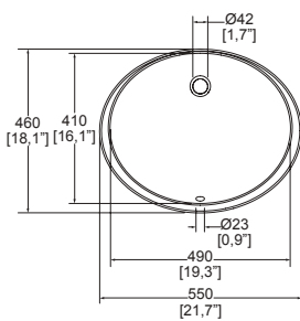
Dimensiones: vista cenital
